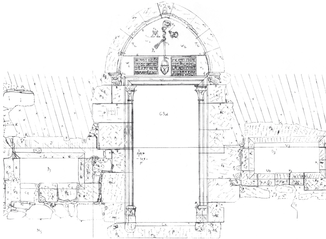
Abbaye de Lagrasse (Aude). Chapelle de l'abbé Auger de Gogenx, porte ouest de la chapelle haute (Relevé et dessin : Andreas HARTMANN-VIRNICH)
